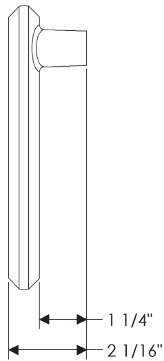
L21075 Long Emile Lever
