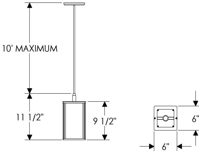
PE465 Echo Pendant 6" x 6" x 131 1/2"
