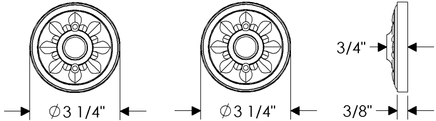
E30803
