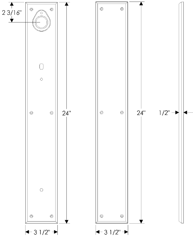
G681
