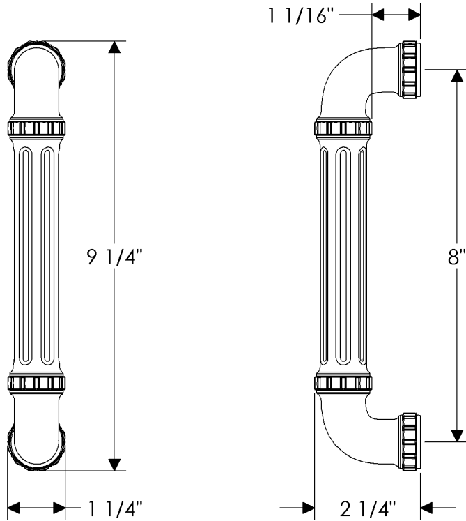
G30167 Pillar Grip
