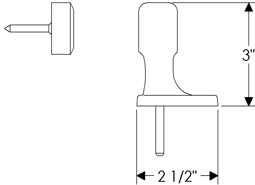
DSH235 Door Stop - Magnetic 2 \frac{1}{2}"
