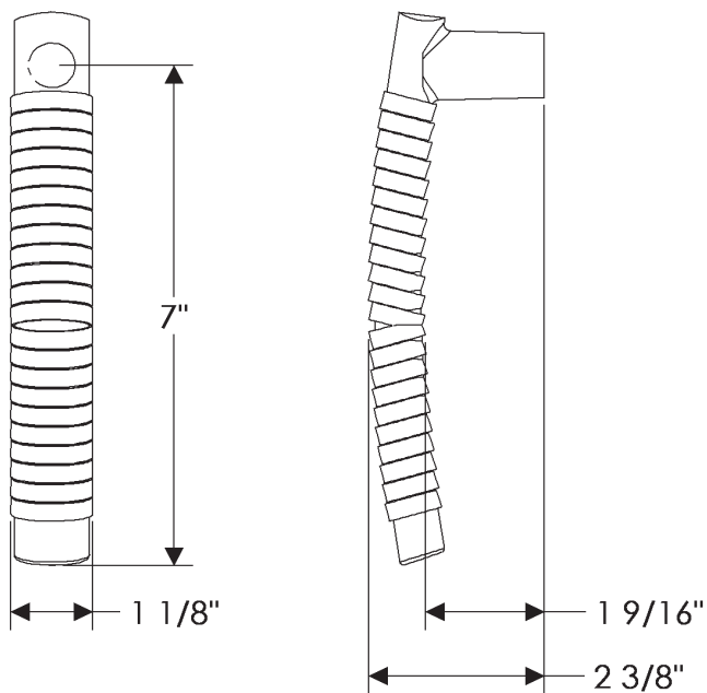
L173 Long Lariat Lever
